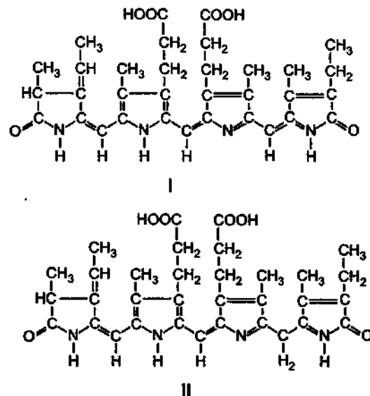
Рис. 170. Структурные формулы фикобилинов: I – фикоцианиобилин; II – фикоэритробилин
